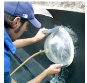
Die Nähte werden zu 100 Prozent mit einer Unterdruck-Saugglocke auf Sicherheit überprüft
